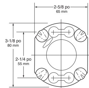
Bride intermédiaire
